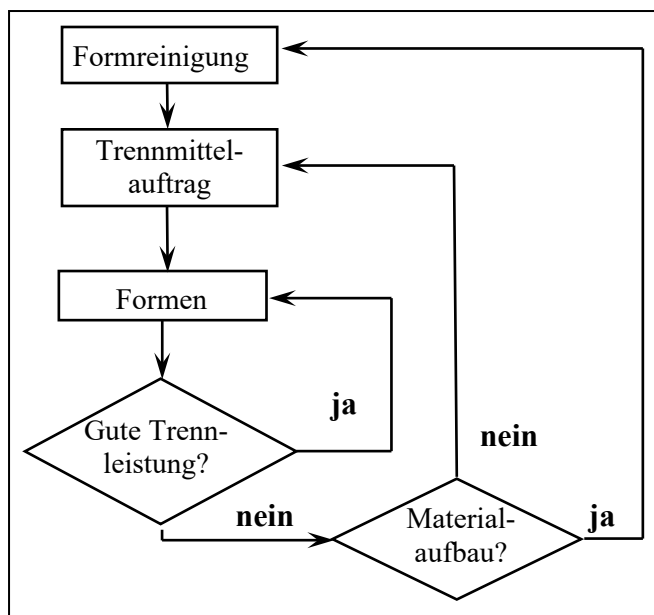
Abbildung 1 Anwendungszyklen von semi-permanenten Trennmitteln in der Gummiproduktion
